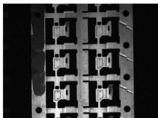
Là encore, la pièce en cuivre brillant n'émet aucun reflet grâce à la BL BAR montée en éclairage directif
