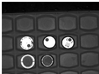
Ici, les reflets des pièces circulaires métalliques sont supprimés
